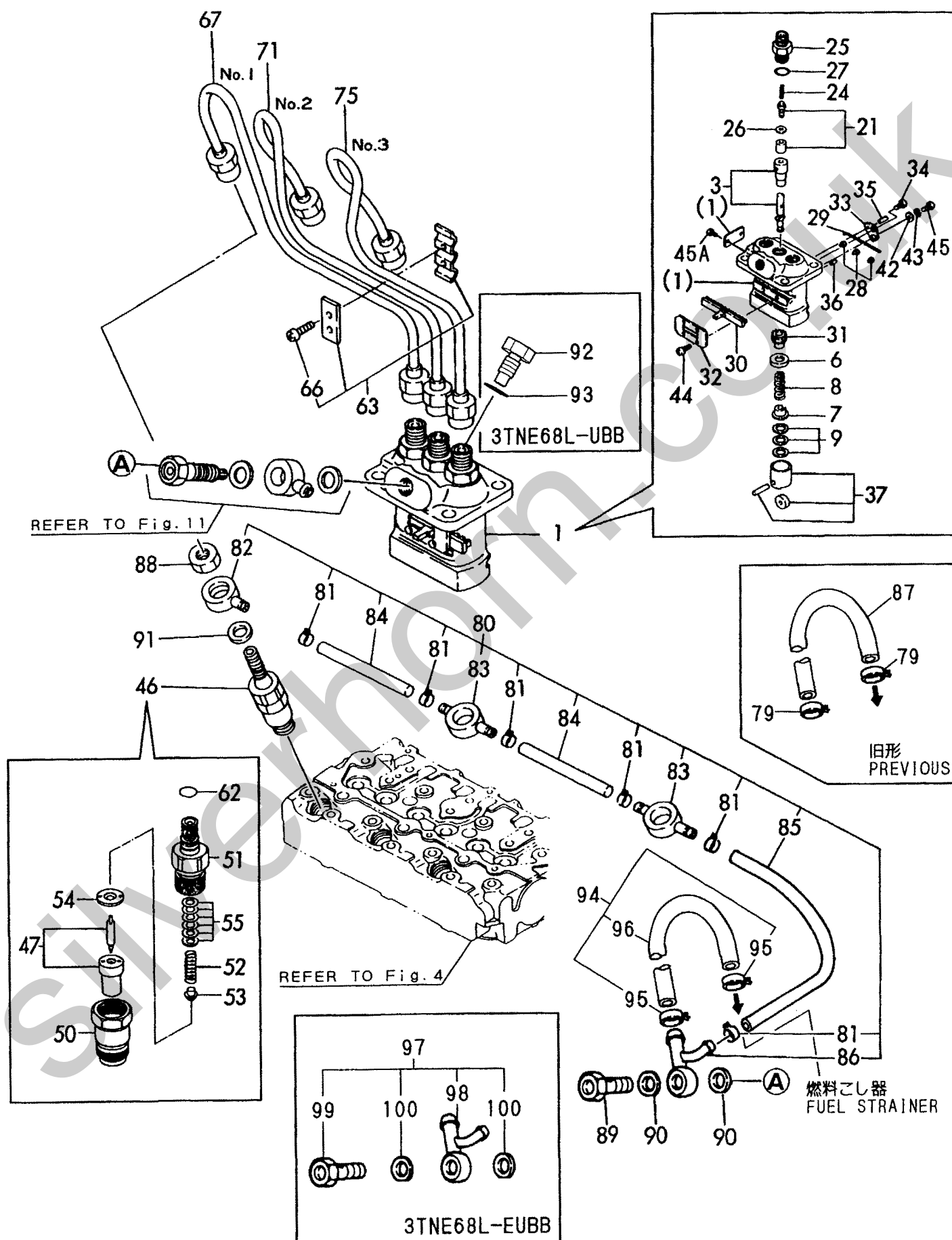
Fig. 10 燃料噴射装置 FUEL INJECTION DEVICE
