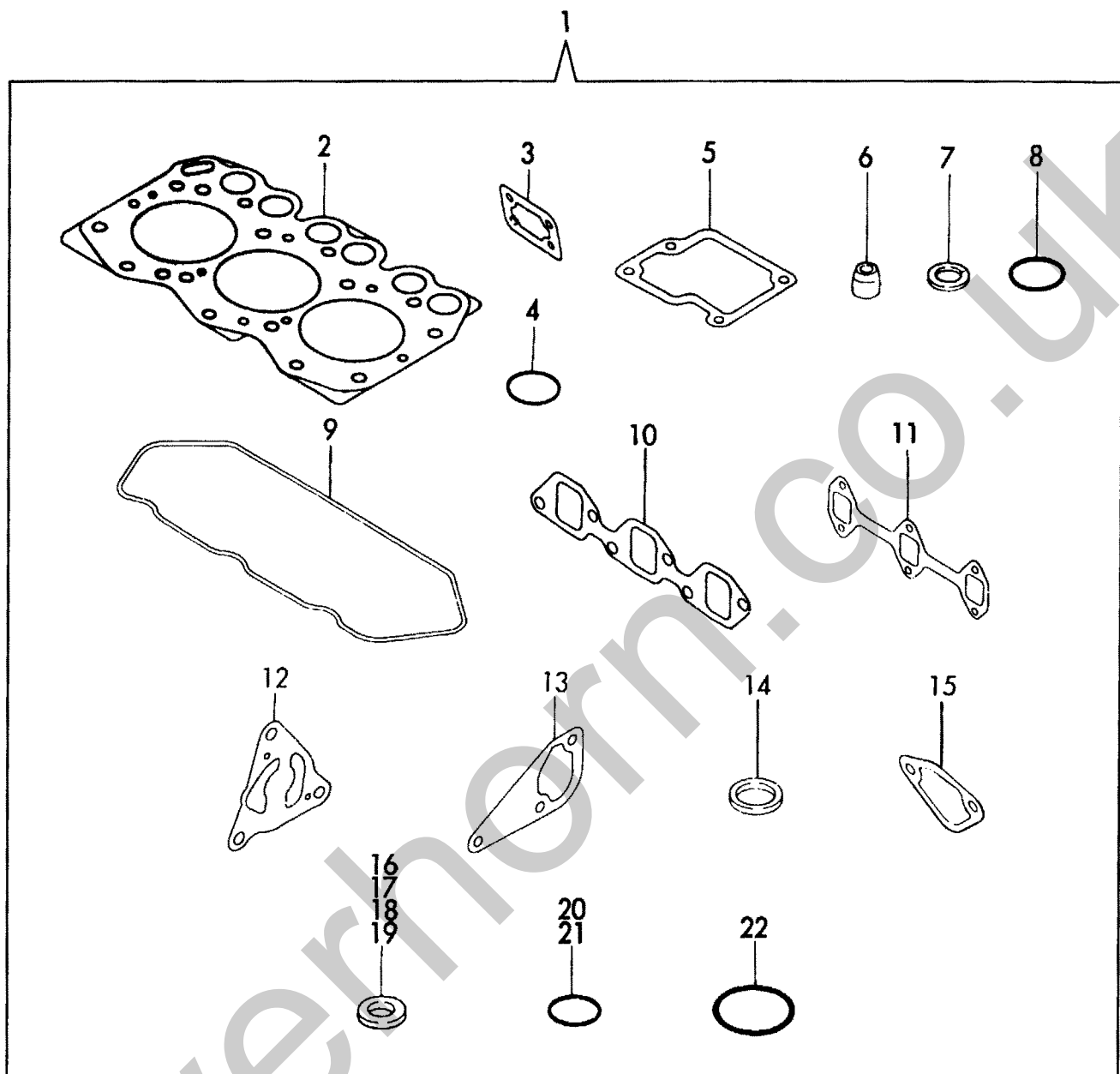
Fig. 15 パッキンセット (オプション) & 工具 GASKET SET (OPTIONAL) & TOOLS
