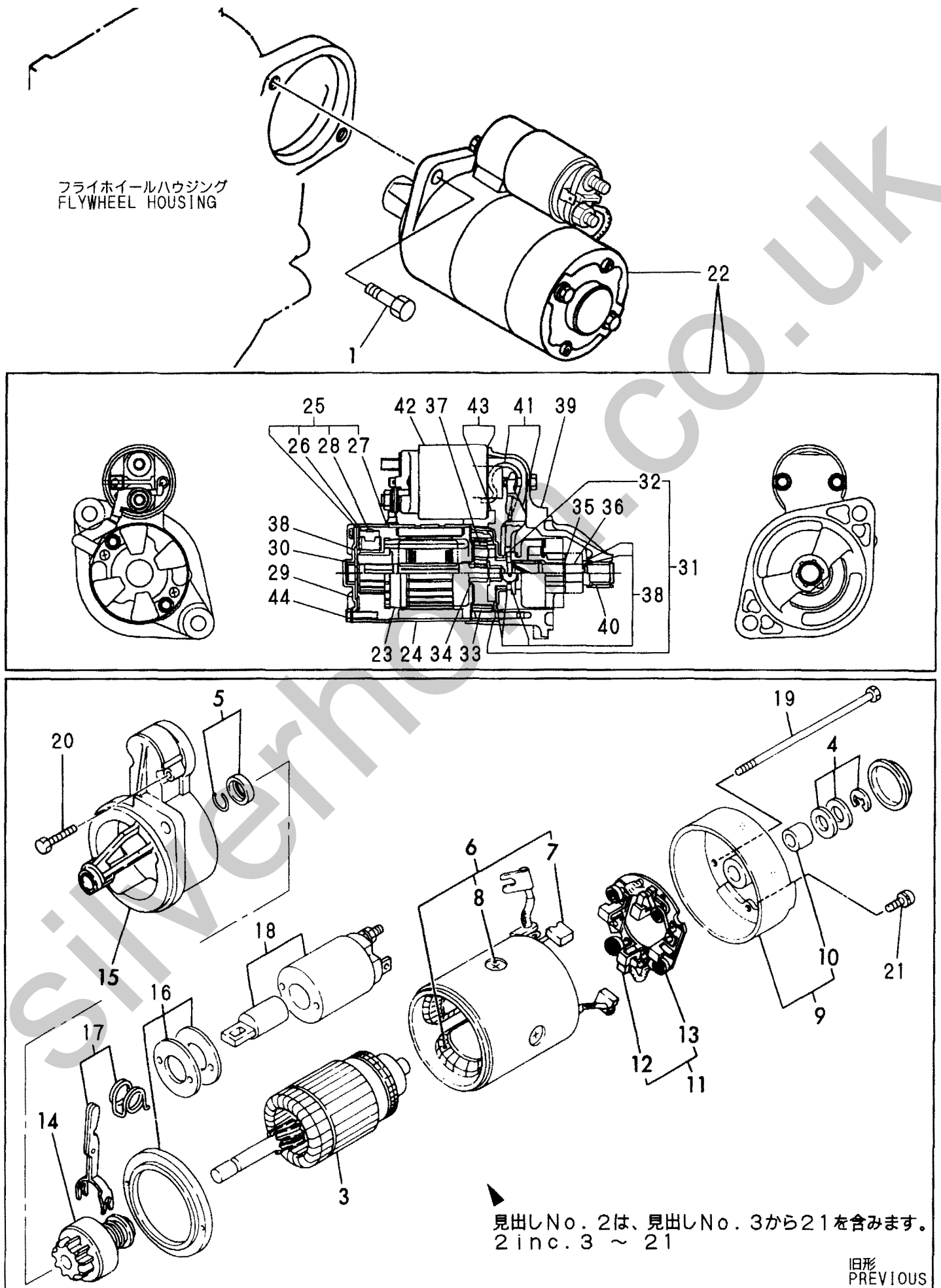
Fig. 13 スターティングモータ STARTING MOTOR
