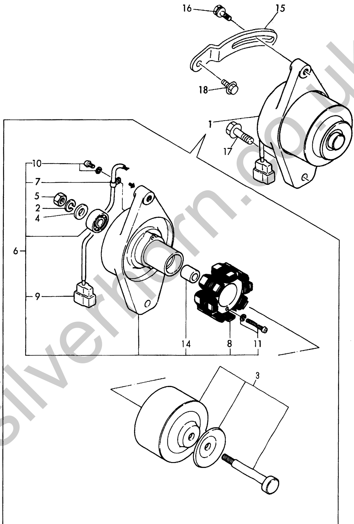
Fig. 14 ジェネレータ GENERATOR
