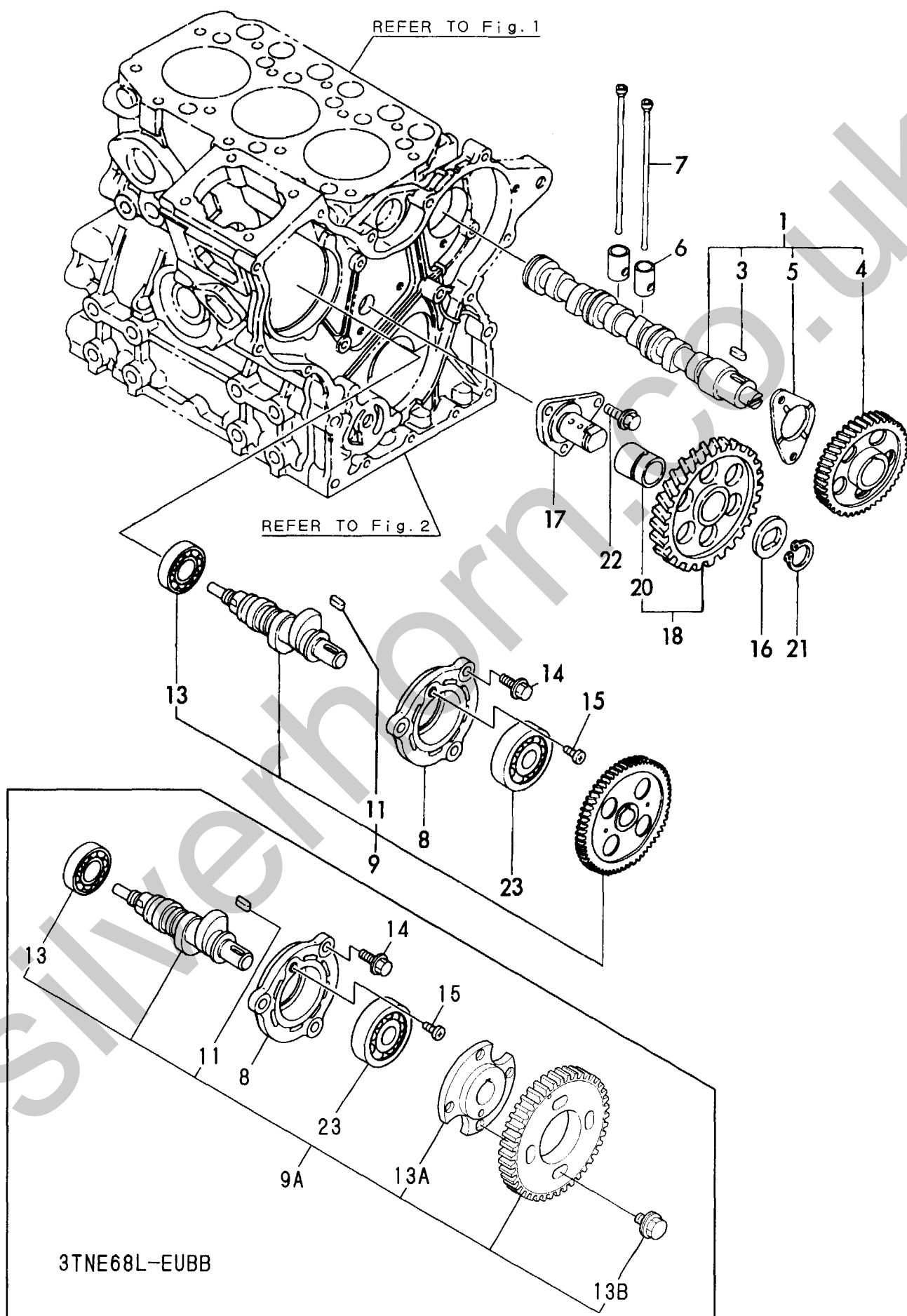
Fig. 6 カムシャフト & 駆動ギヤ CAMSHAFT & DRIVING GEAR
